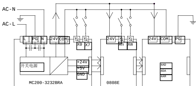
交流电源及辅助电源连接示例
